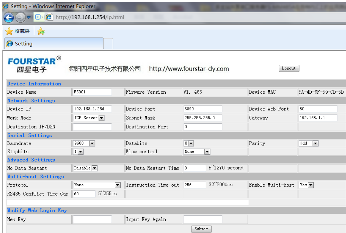
图 1-2 FS-ETH-FP0 参数设置截图
