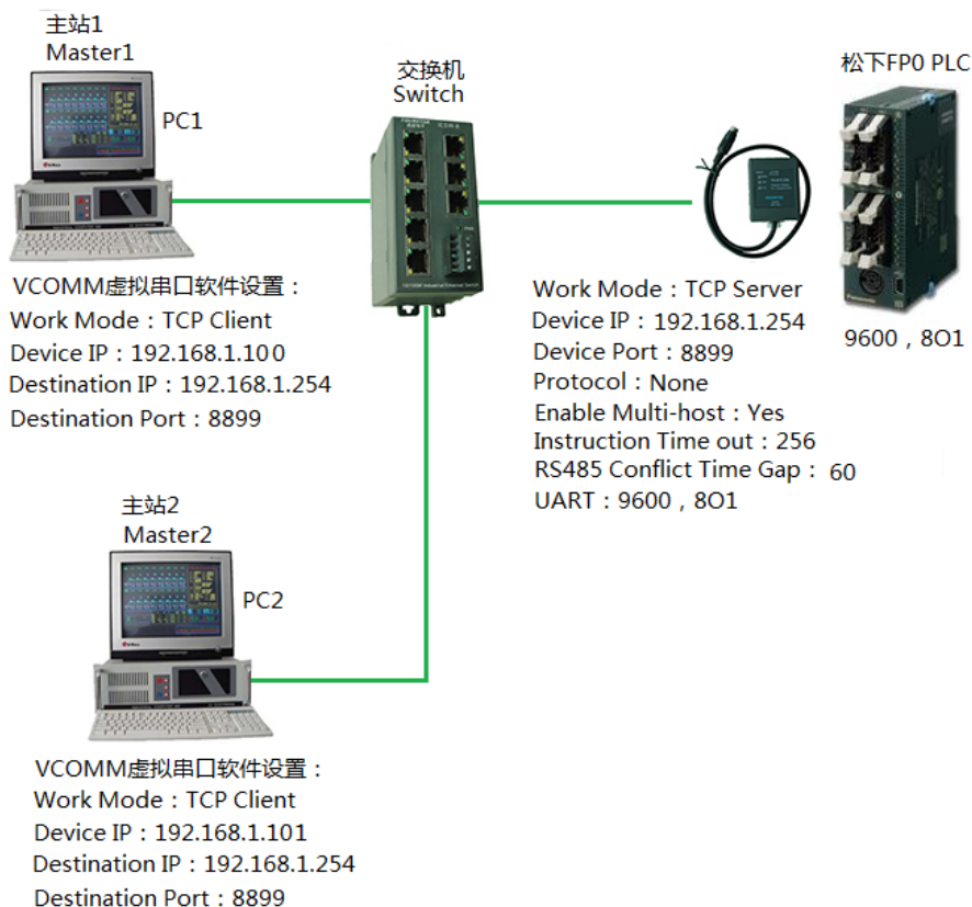
图 1-1 组态王与松下 FP0 系列 PLC 多主站通讯连接拓扑
