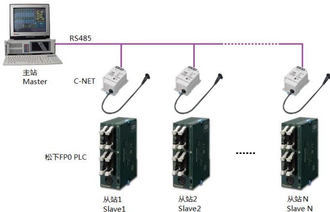
图 1-1 典型的单个主站 RS485 通讯网络拓扑
