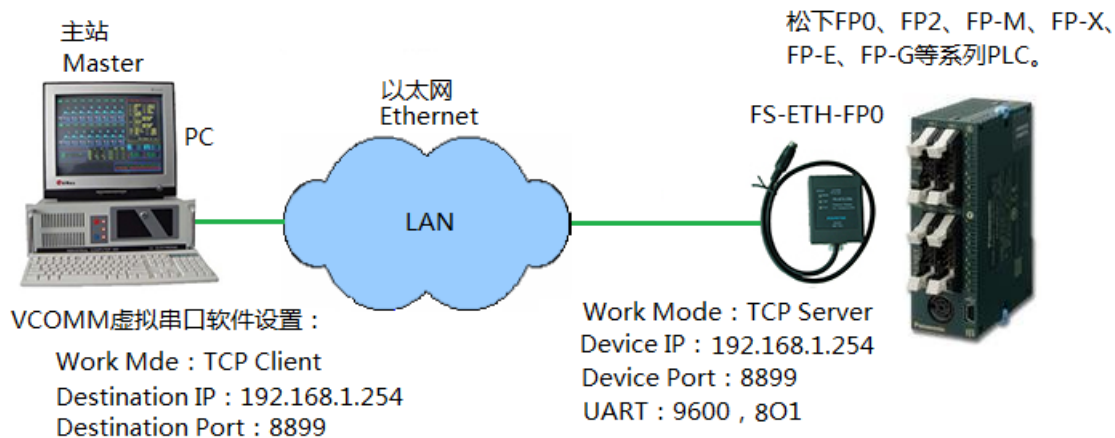
图5.1-1 计算机与松下PLC通过以太网通讯
