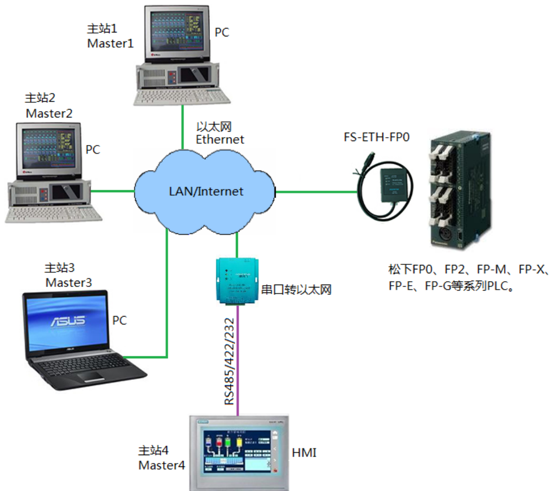
图 1-2 采用 FS-ETH-FP0 的多主站通讯网络拓扑
