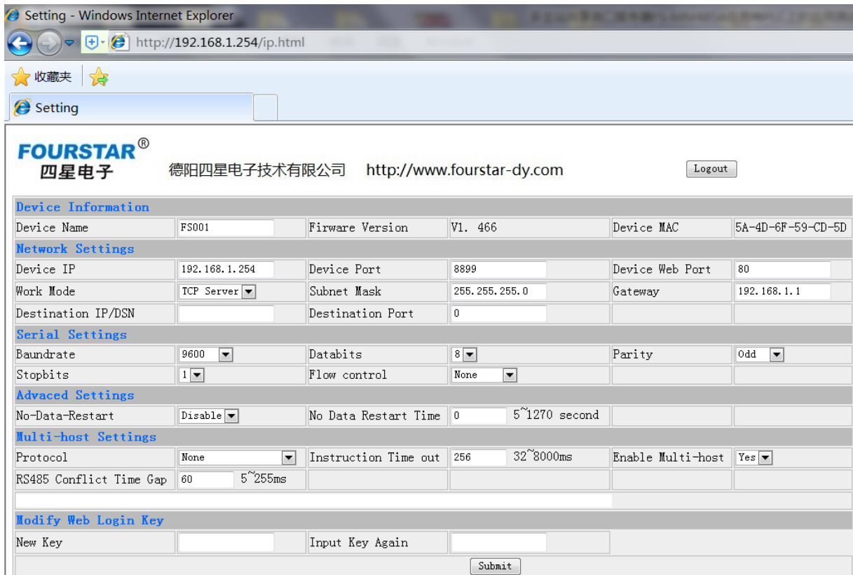
图5.2-1 FS-ETH-FP0作多主站共享串口服务器时的设置
