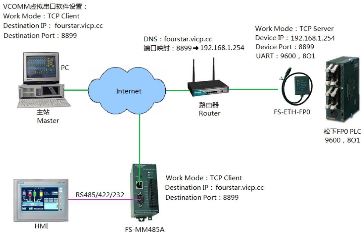
图5.3-1 FS-ETH-FP0在互联网上的通讯网络拓扑
